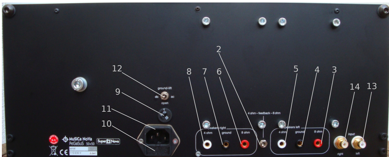
Rückansicht PeGaSuS 50/50
